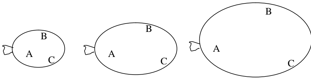
Gambar 6.2 Balon karet yang ditiup. Titik A, B, dan C pada permukaan balon karet apabila ditiup akan saling menjauh.
