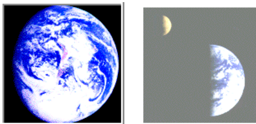
Gambar 6.12 Permukaan Bumi
