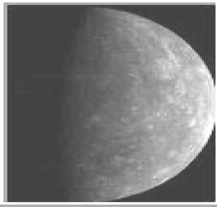
Gambar 6.10 Planet Merkurius
