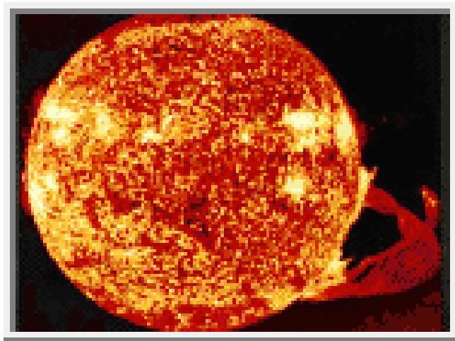
Gambar 6.4 Matahari
