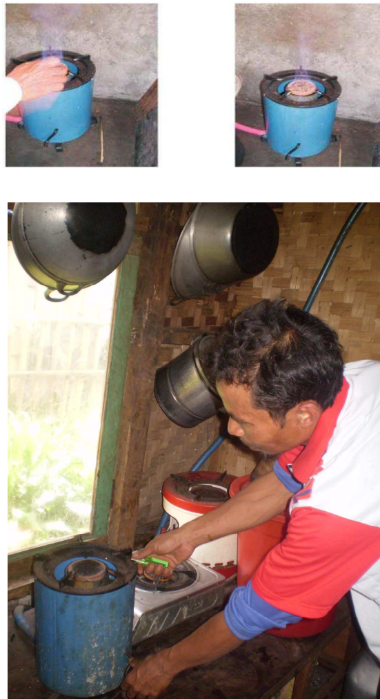
Gambar 8 Pengoperasian Kompor Biogas
