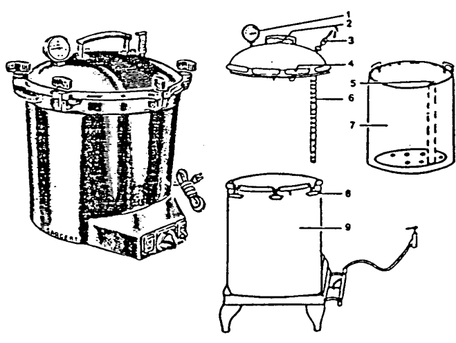
GAMBAR 2-2. Sterilisator uap portable disertai sketsa yang menunjukkan bagian-bagian alat tersebut.
