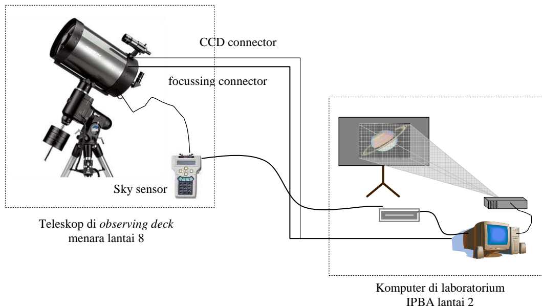
Gambar 1 Skema jaringan optimalisasi teleskop Schmidt Cassegrain Celestron.
