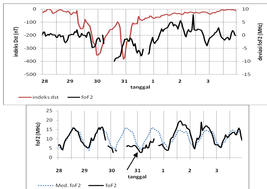
Gambar 1. Variasi indeks Dst terhadap deviasi foF2 pada rentang waktu 28 Oktober–3 November 2003 ( atas ). Variasi nilai foF2 (garis penuh) terhadap mediannya (garis putus-putus). Nilai foF2 pada grafik bernilai negatif. Tanda panah menunjukkan kejadian badai ionosfer negatif ( bawah ).
