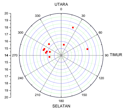
Gambar 3. Grafik V_{sky} terhadap azimut.
