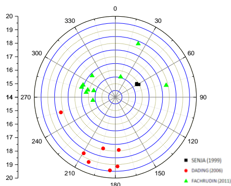
Gambar 5. Diagram polar kecerahan langit Observatorium Bosscha FMIPA ITB dari ketiga pengukuran terhadap azimut.
