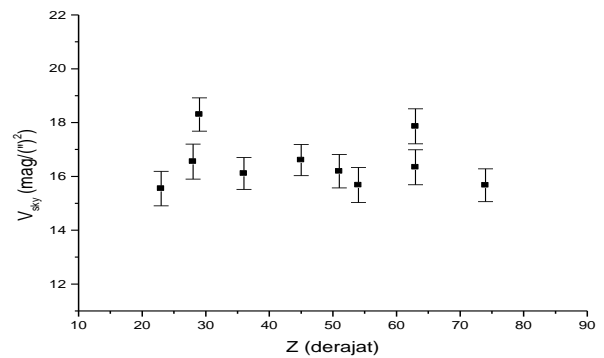
Gambar 2. Grafik V_{sky} terhadap jarak zenit ( z ).
