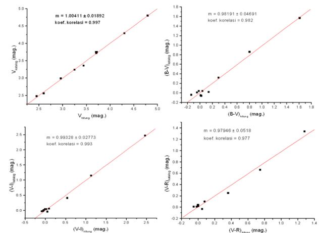
Gambar 1. Grafik magnitudo perhitungan terhadap magnitudo standar katalog.
