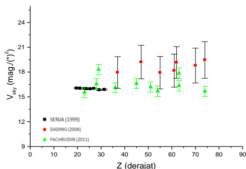
Gambar 4. Grafik kecerahan langit Observatorium Bosscha FMIPA ITB dari ketiga pengukuran terhadap jarak zenit
