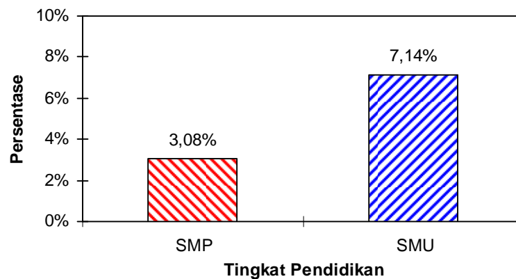
Gambar 1. Persentase materi IPBA di pelajaran fisika dalam kurikulum 2004 untuk sekolah menengah
