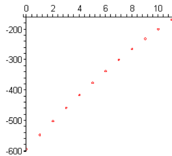
Gambar 6. Grafik Kontrol u(k)
