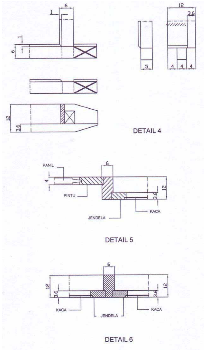
Gambar.23 Detail konstruksi Kosen pintu dan Jendela
