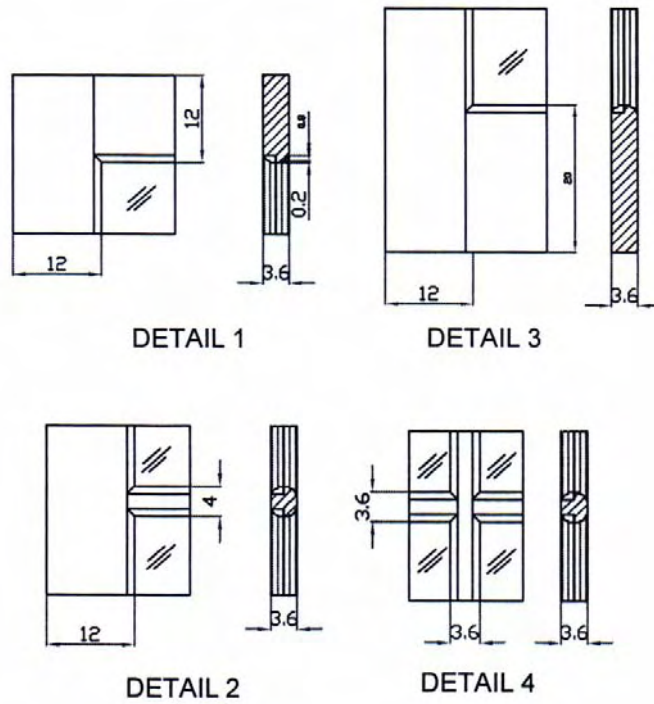
Gambar.25 Konstruksi Pintu Kaca
