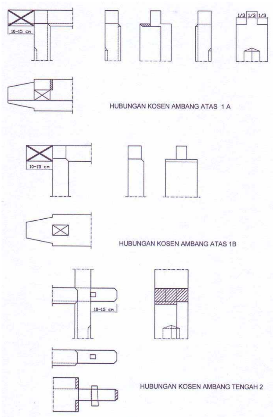
Gambar 2 Detail Hubungan Konstruksi Kosen Pintu
