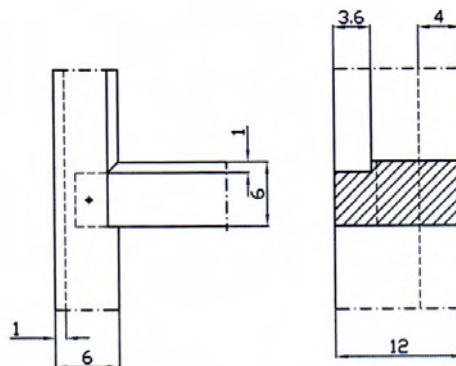
KOSEN PINTU TUNGGAL
