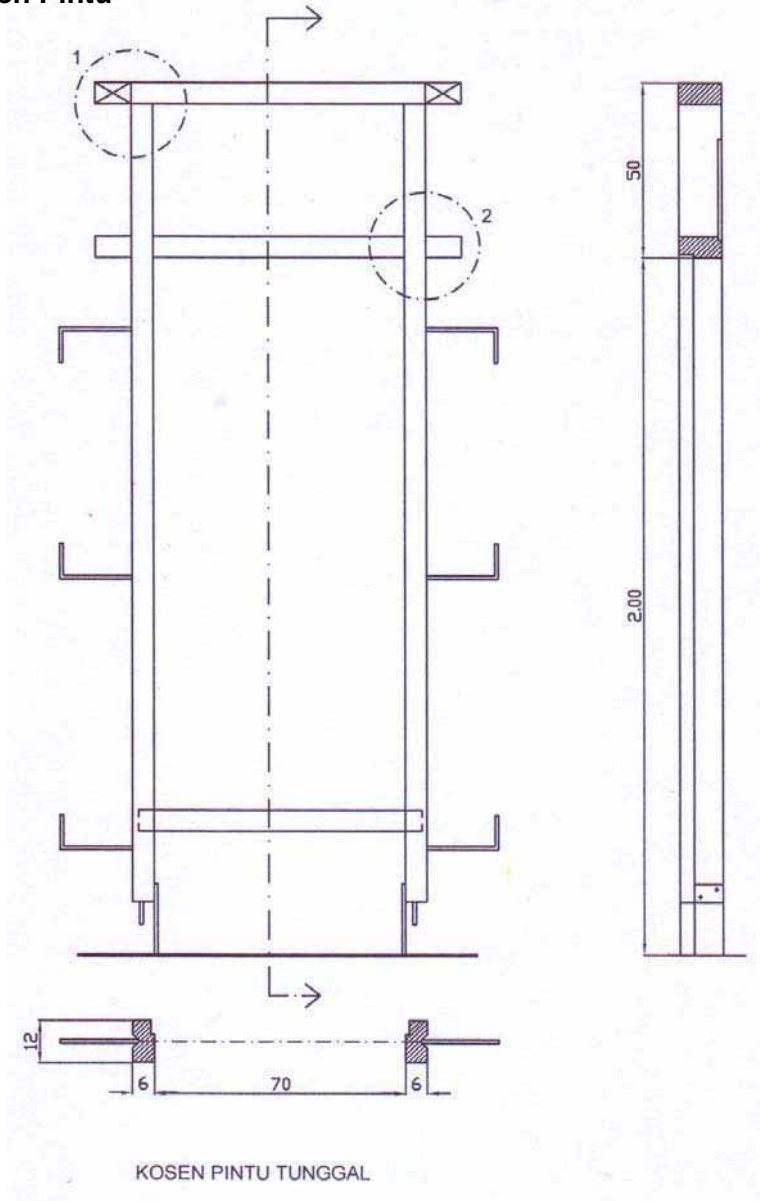
Gambar 1 Kosen Tunggal
