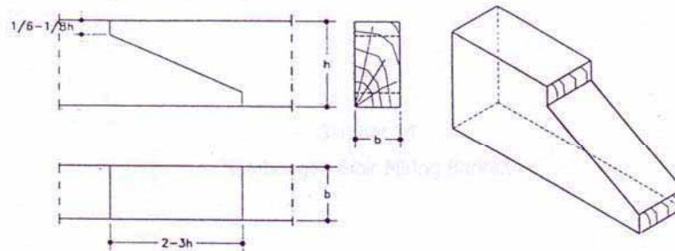
Sambungan Bibir Miring Berkait
