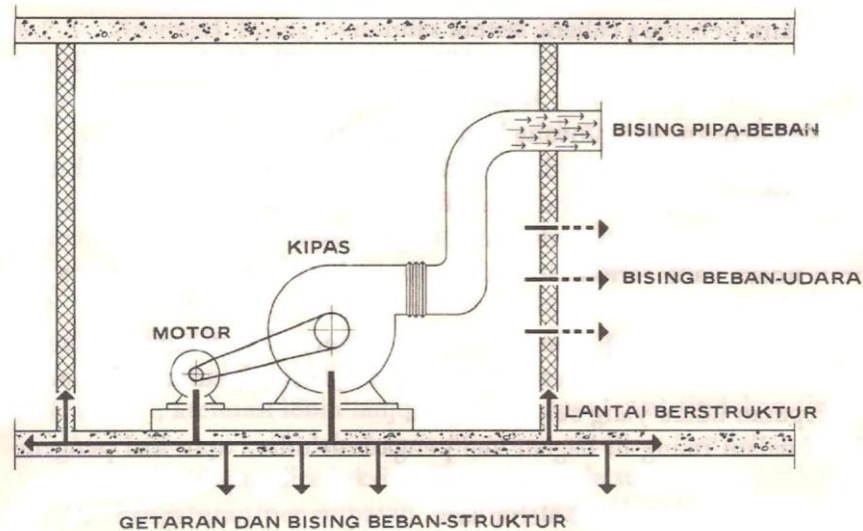
Sumber-sumber bising utama pada system pengaturan udara
