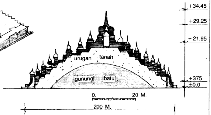
Potongan dari ②
