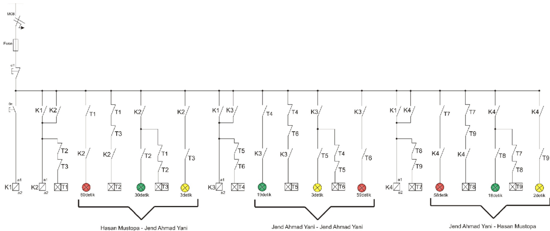
Gambar instalasi traffic light menggunakan 4 kontaktor
