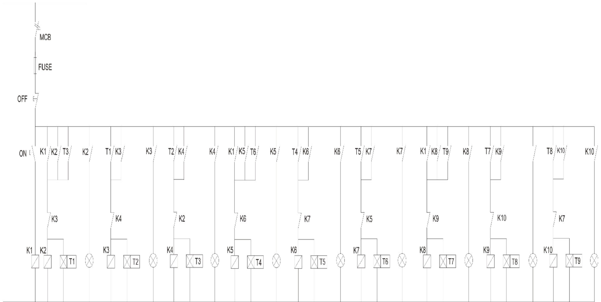
Gambar instalasi traffic light menggunakan 10 kontaktor
