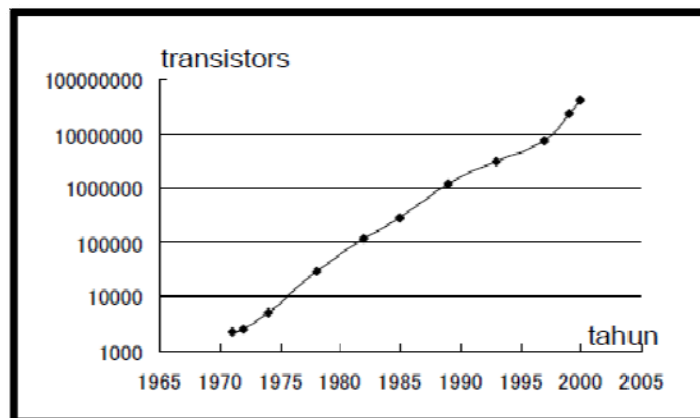
Gambar 1. Perkembangan jumlah transistor pada IC dari tahun ke tahun yang menunjukkan kesesuaian dengan Moore's law.
