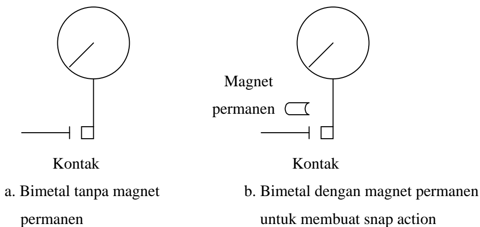
Gambar 14. Bimetal dengan magnet permanen
