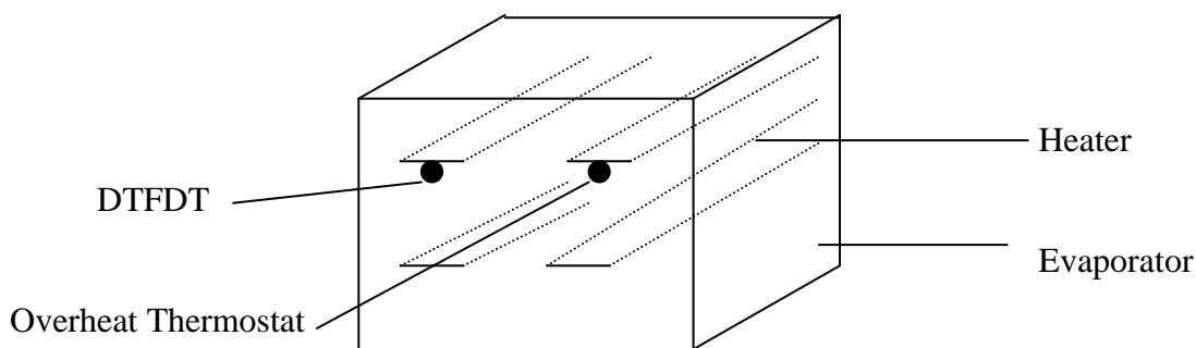
Gambar 9. Penempatan DFTD Thermostat
