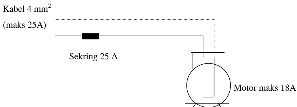
Gambar 2. Instalasi ukuran kabel dan kekuatan sekering
