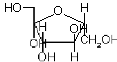
D-Fructose
