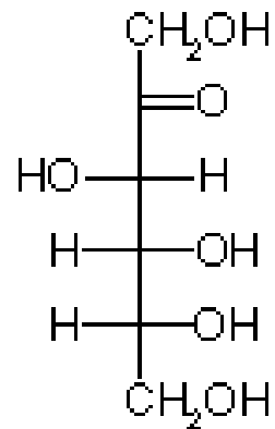
D-Fructose
