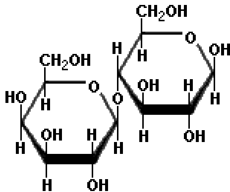
Lactose
