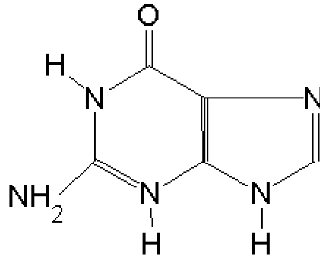
Guanin
