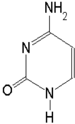
Cytosin
