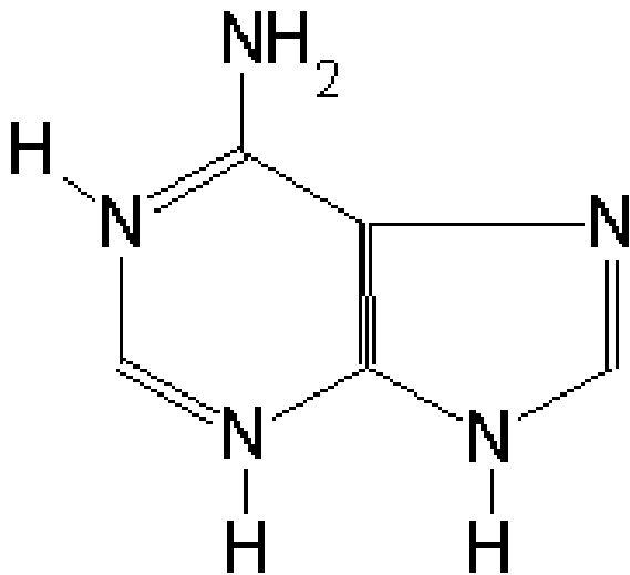
Adenin
