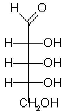
D-Ribose
