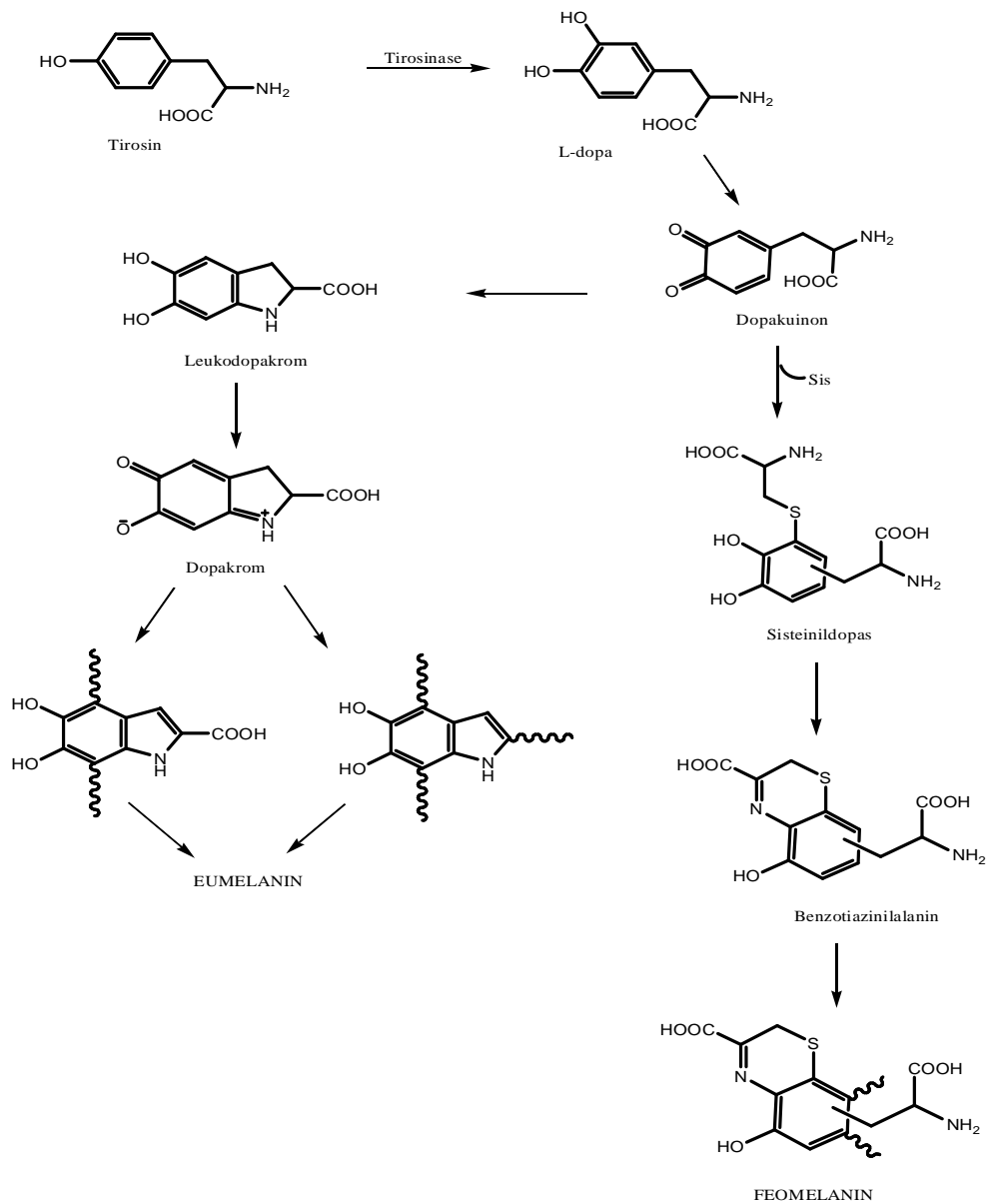
Gambar 2. Biosintesis melanin (Prota dkk. (1988) di dalam Jacques (tanpa tahun))
