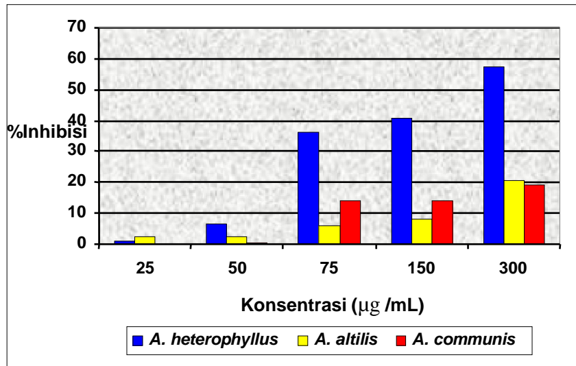
Gambar 1. Inhibisi ekstrak metanol kulit batang A. heterophyllus (nangka), A. altilis (sukun) dan A. communis (kluwih) pada konsentrasi 25, 50, 75, 150 dan 300 µg/mL.
